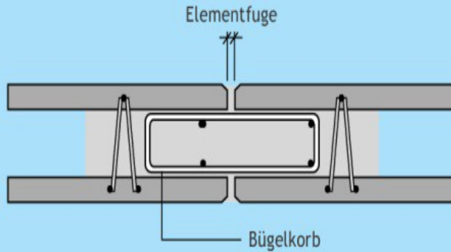
Horizontalschnitt Wand
