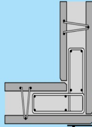
Horizontalschnitt Ecke
